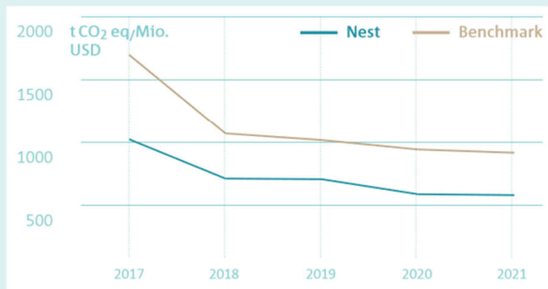
CO 2 -Absenkung Nest-Aktien Portfolio 2017–2021
