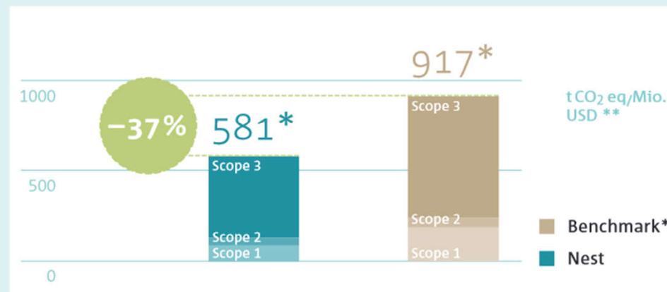
CO 2 -Intensität Nest-Aktien Portfolio per 31.12.2021
